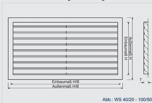
Rechteckige Ausführung
