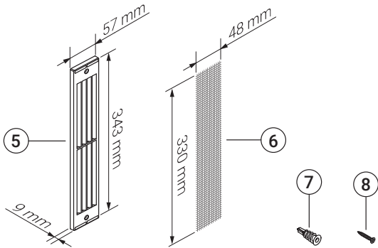
Laibungsgitter Kunststoff Reveal grille plastic
