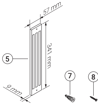
Laibungsgitter Metall Reveal grille metal
